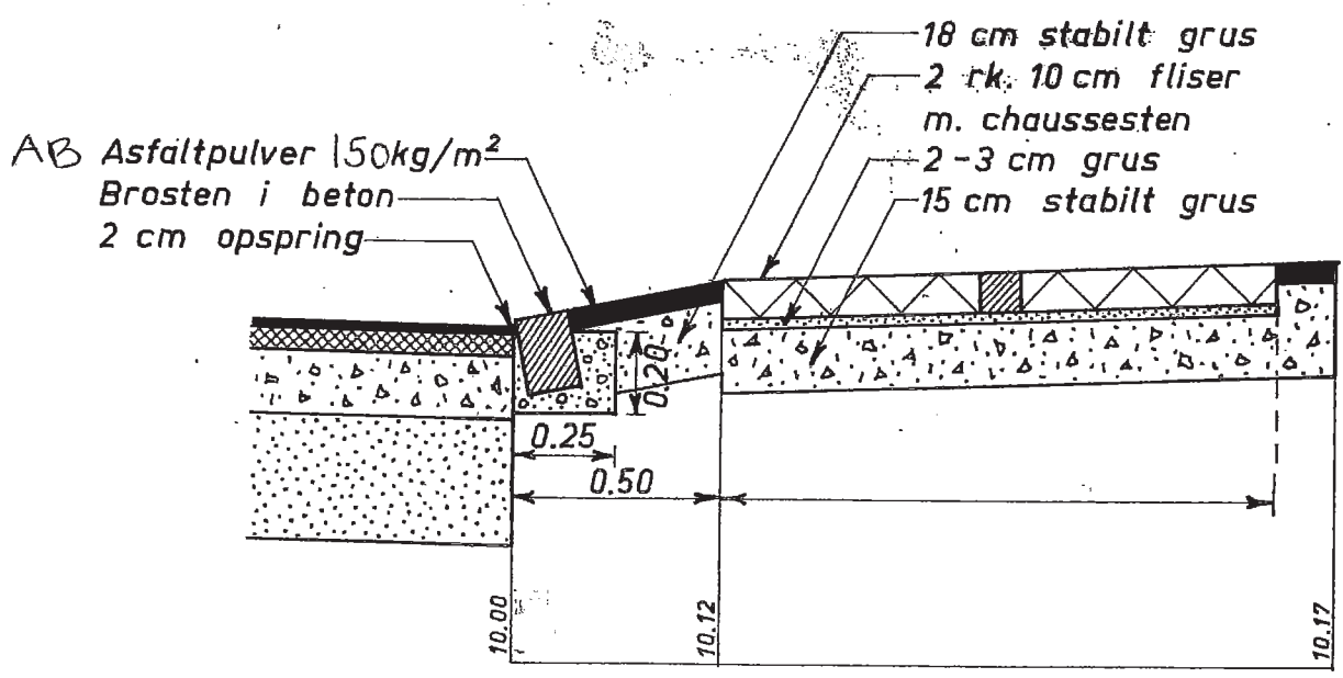
Snit, 1:20
