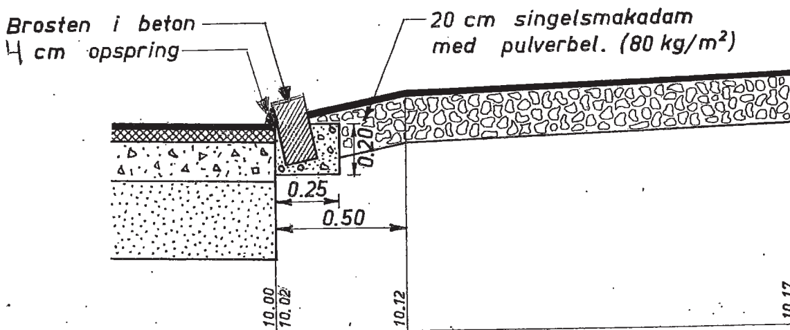
Snit, 1:20
