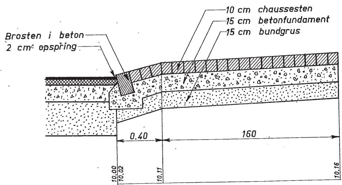
Snit, 1:20
