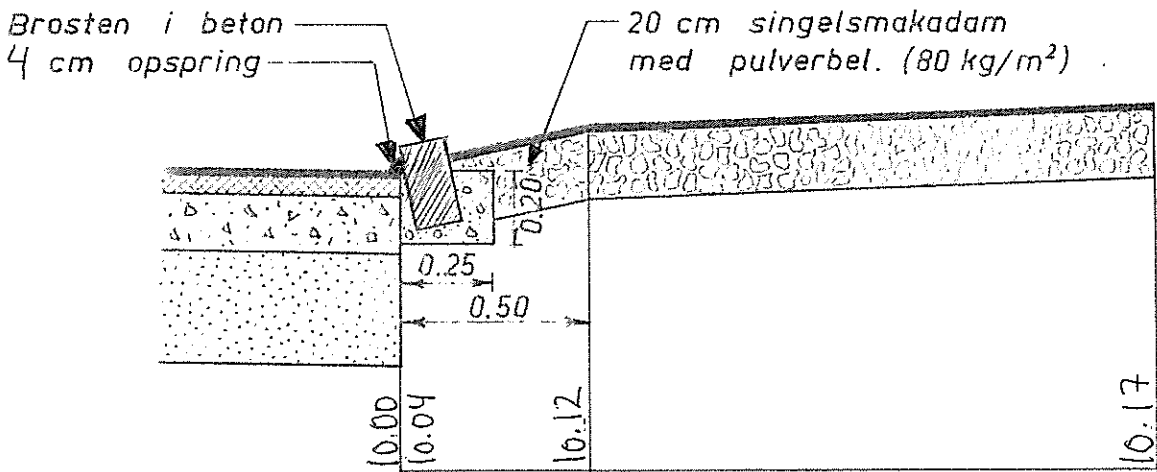
Snit, 1:20
