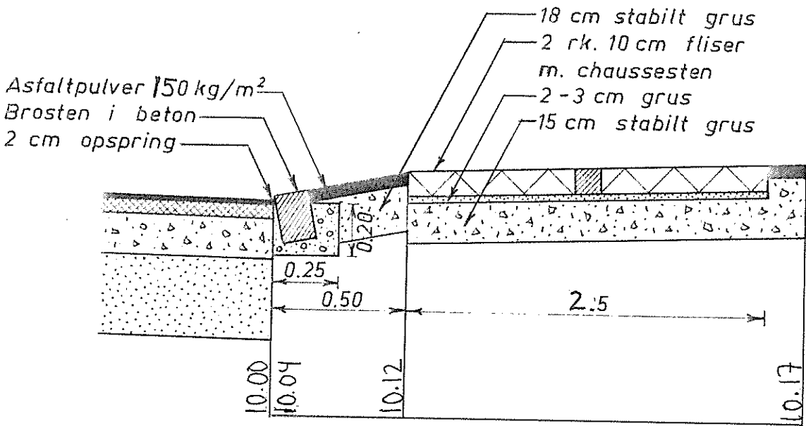
Snit, 1:20
